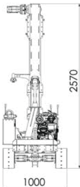
Pogled sa zadnje strane – MINIMALNA VISINA
