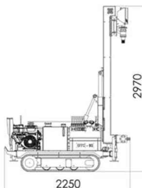
Pogled sa strane - MAKSIMALNA VISINA
