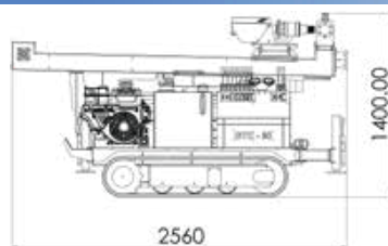
Pogled sa strane - MAKSIMALNA VISINA
